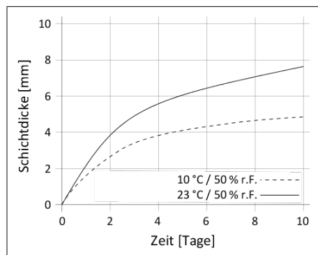
Diagramm 1: Durchhärtageschwindigkeit Sikaflex®-522
