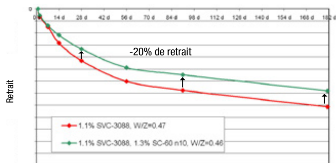
Essai in situ 300 kg CEM II A-LL 42,5 0/32 mm Durée en jours
